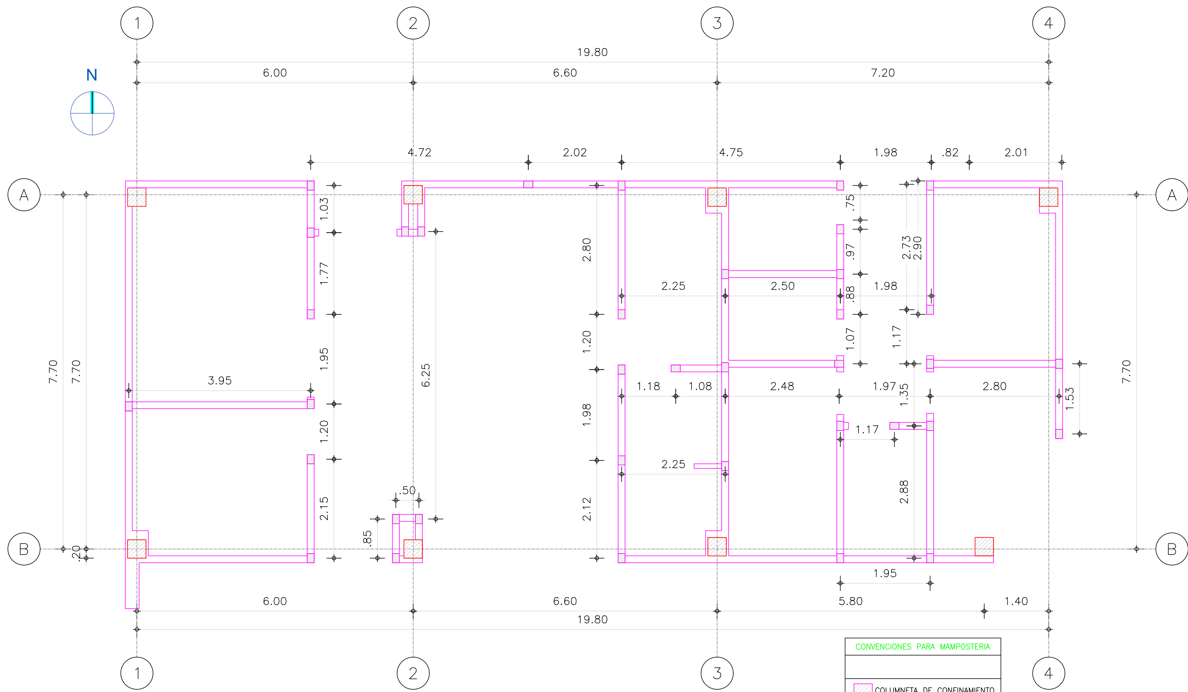
PLANTA DE CONFINAMIENTOS PARA MUROS Ó REFUERZOS DE DOVELAS MODULO ESTRUCTURAL 1 1 : 50
